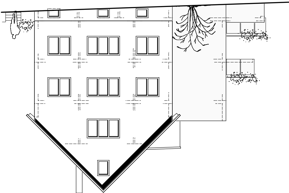
Süd-Ost Ansicht M 1:100
